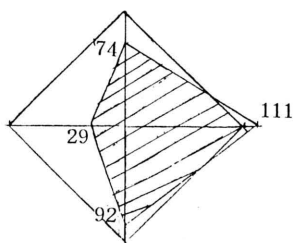
園部町
